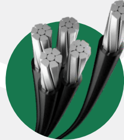
Özünü saxlayan, izolyasiya olunmuş, hava elektrik veriliş xətləri
